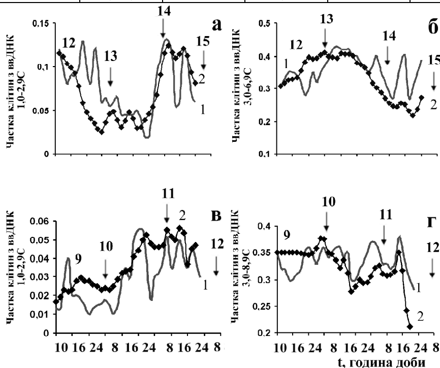
Рис. 1. Динаміка зміни частки субпопуляцій клітин з ввДНК 1,0–2,9С (а) та 3,0–6,9 С (б) у варіанта К-27(10С) протягом 12–15-ї дб культивування (1 — потік I_l(t) , визначений з експерименту; 2 — потік I_l(t) , визначений з рівняння, l=1,2 ) і субпопуляцій клітин з ввДНК 1,0–2,9С (в) та 3,0–8,9 (г) у варіанта К-27(Рж) протягом 9–12-ї дб культивування (1 — потік I_l(t) , визначений з експерименту; 2 — потік I_l(t) , визначений з рівняння, l=1,2 ). Всі дані згладжено за середнім змінним. Стрілками позначено початок відповідної доби росту
